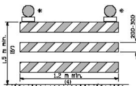
TYPE III BARRICADE
