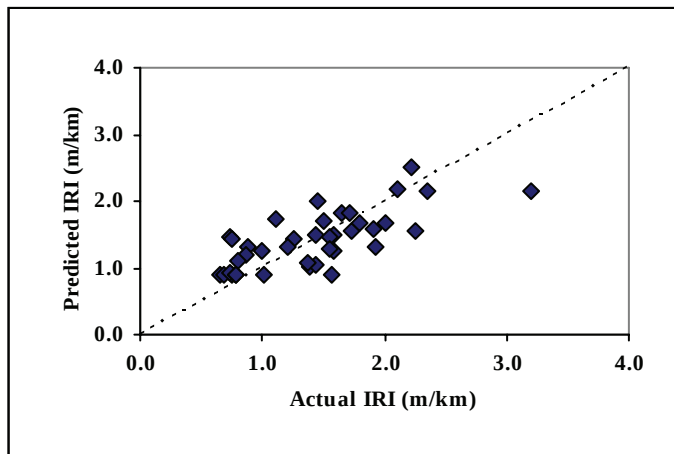
Figure 3. Actual versus predicted values of IRI
