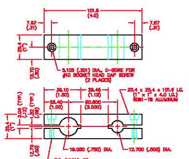
2 LVDT HOLDER
